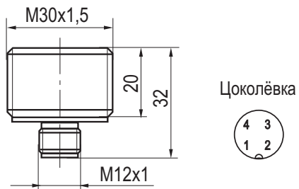
Габаритный чертеж
